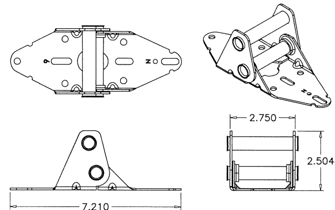
#6 HINGE (11 GA. STEEL)
